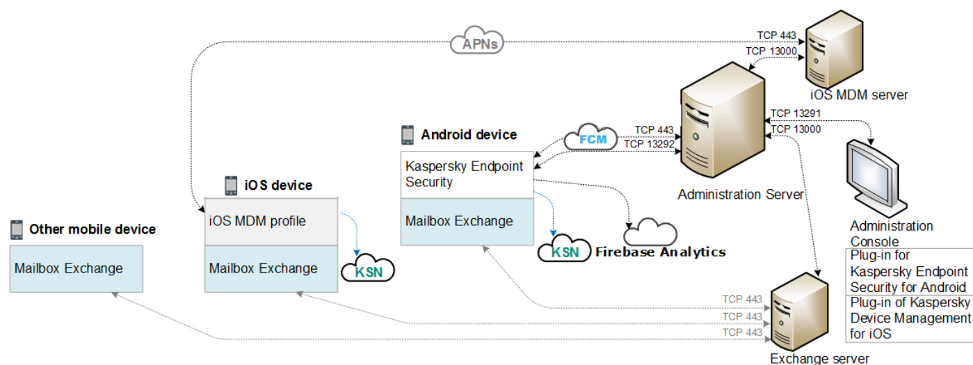
Архитектура Kaspersky Security для мобильных устройств
