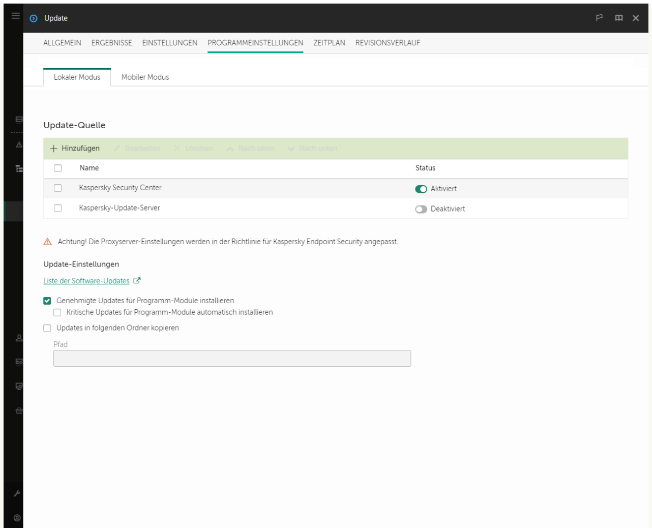
Update-Quellen
