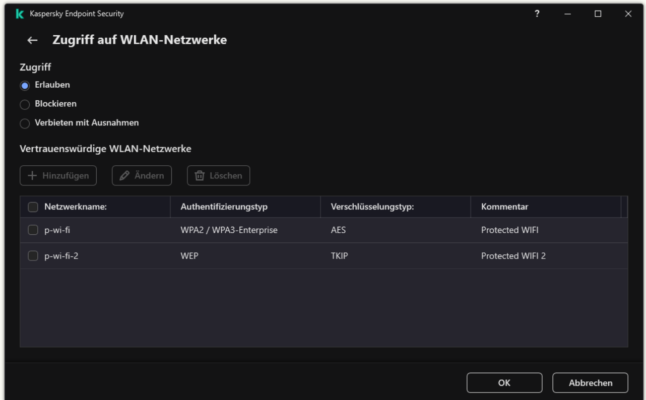
WLAN-Zugriffseinstellungen
