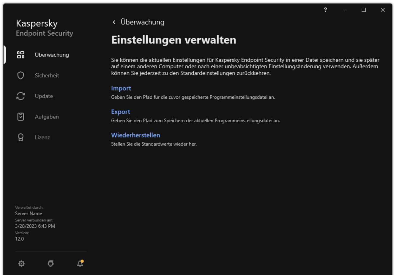
App-Einstellungen verwalten
