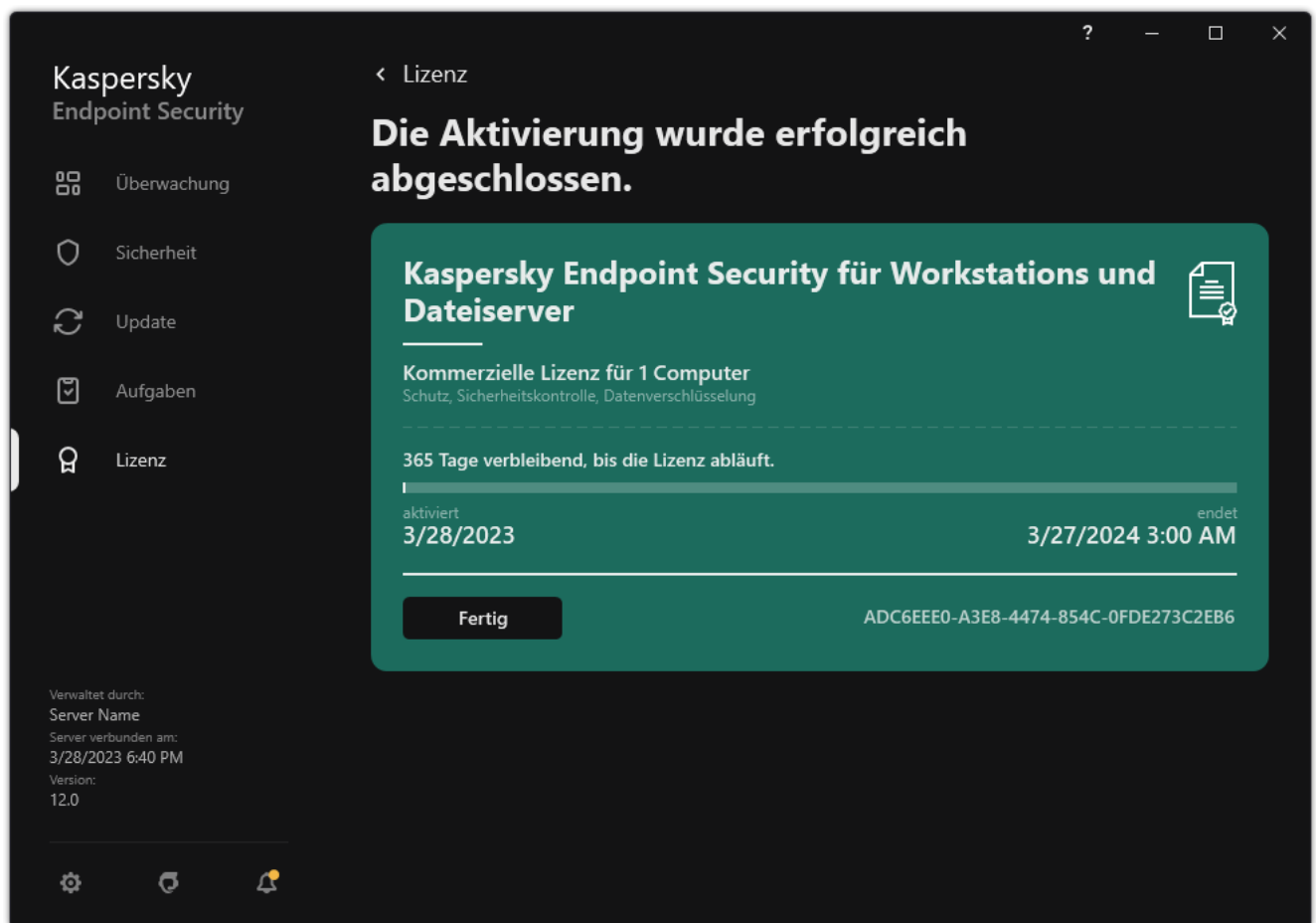
Fenster Lizenzverwaltung
