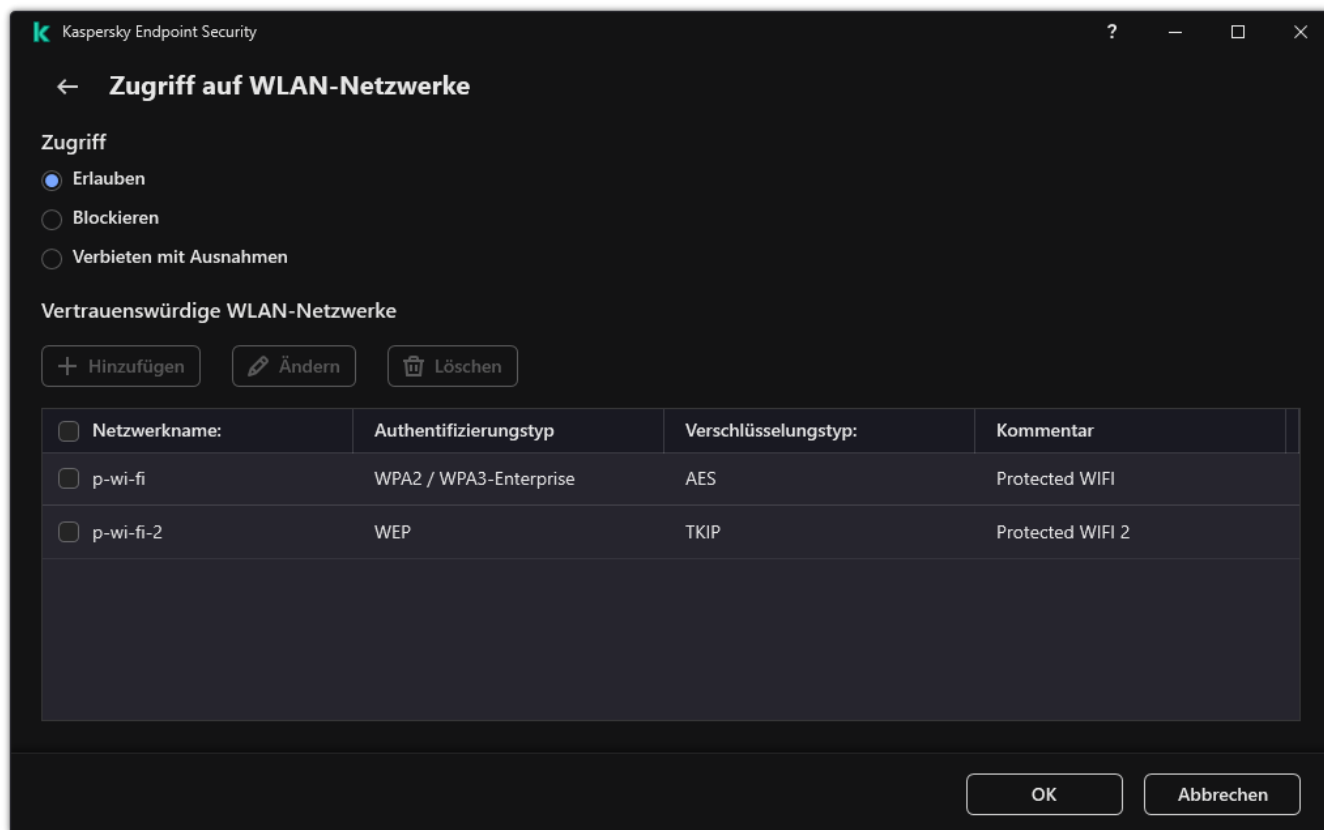
WLAN-Zugriffseinstellungen
