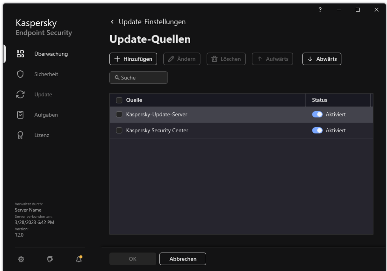
Update-Quellen
