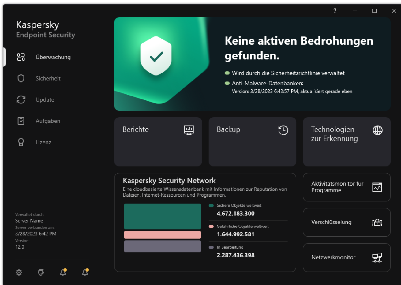
Programmhauptfenster
