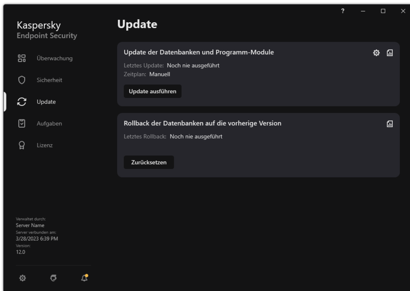
Lokale Update-Aufgaben
