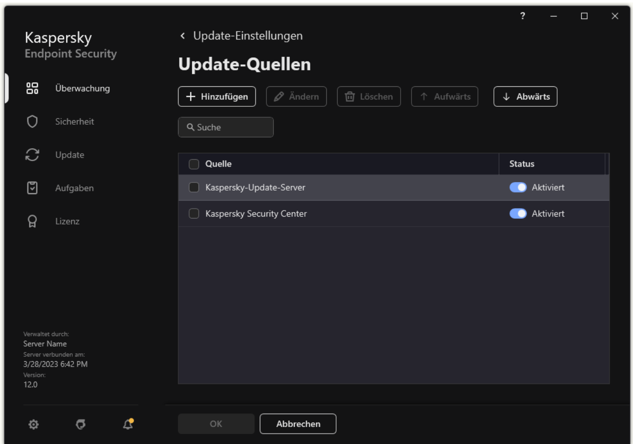
Update-Quellen
