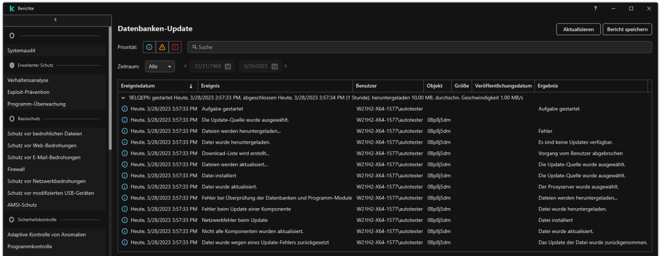
Berichte
