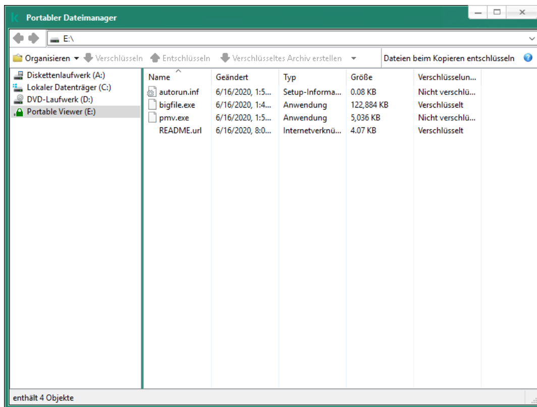
Portabler Dateimanager
