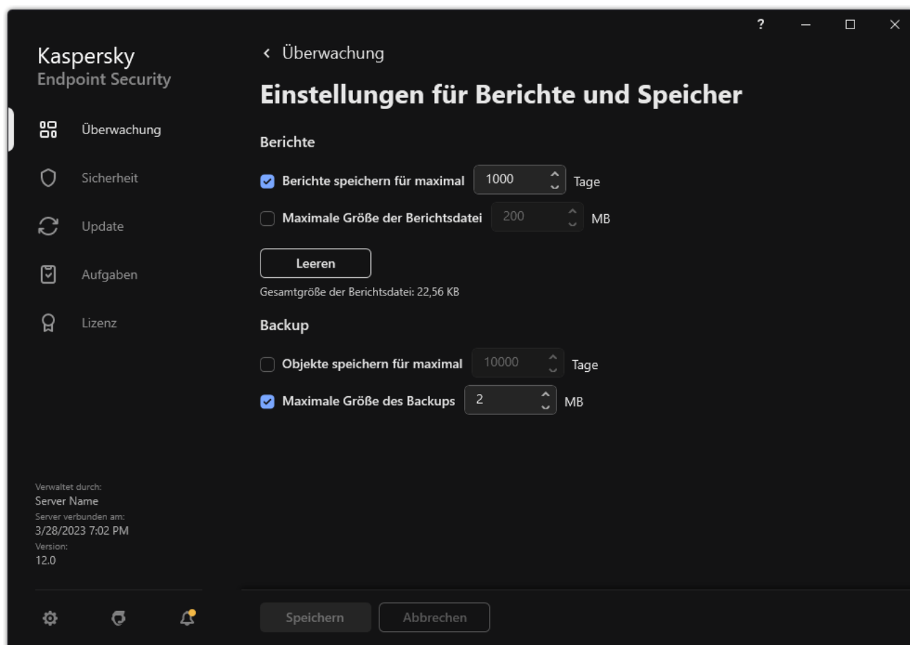
Sicherungseinstellungen
