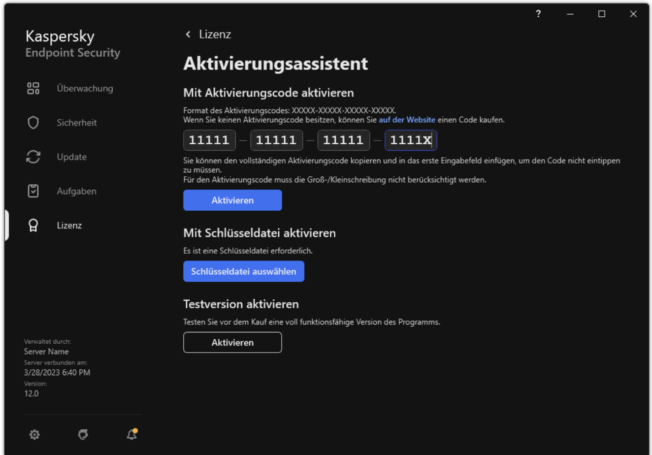
Programm aktivieren
