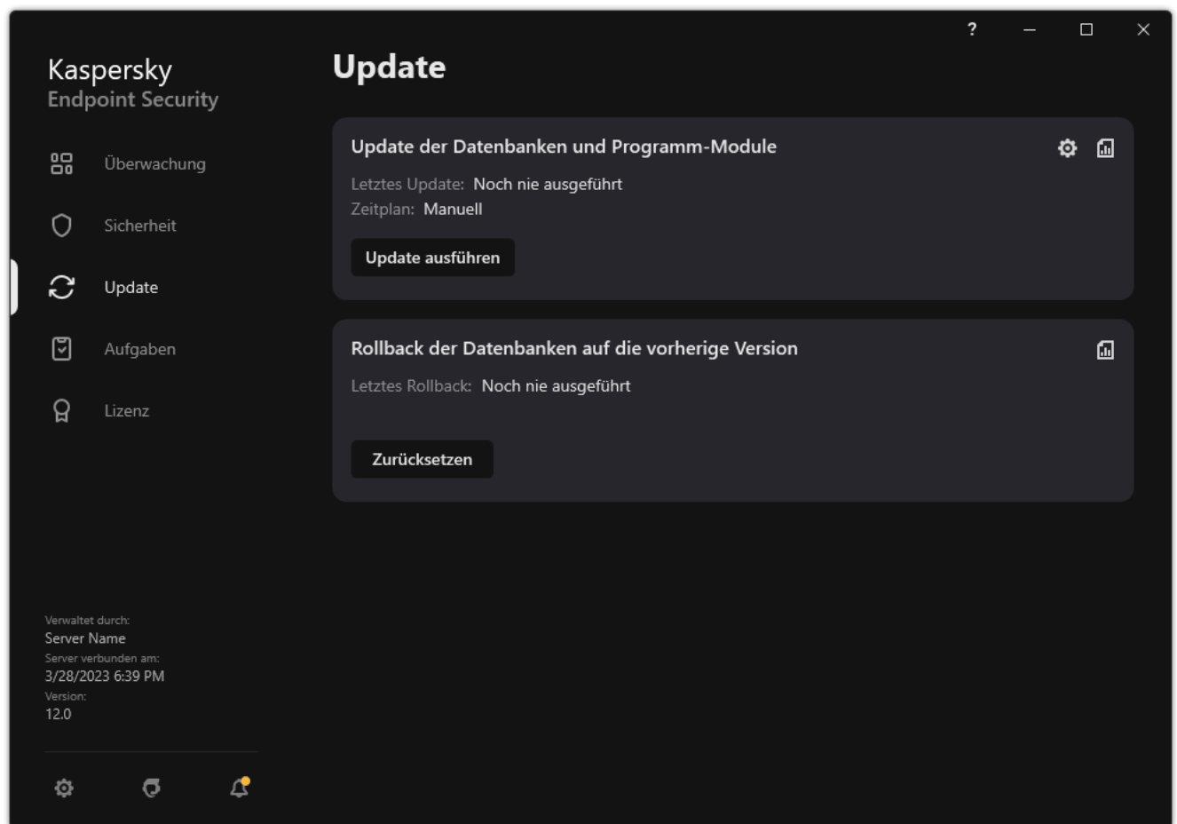
Lokale Update-Aufgaben
