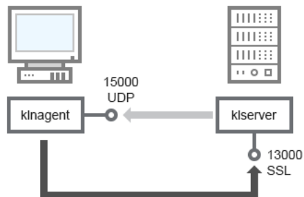
Administrationsserver und Client-Gerät: Verwaltung der Sicherheitsanwendungen, Verbindung über Port 13000 (empfohlen)
