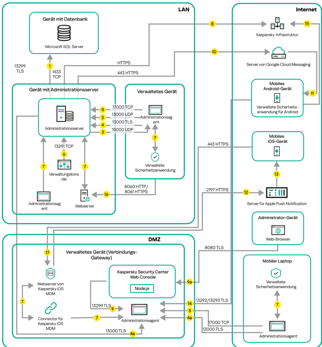
Verwaltete mobile Geräte, die über ein Verbindungs-Gateway mit dem Administrationsserver verbunden sind
