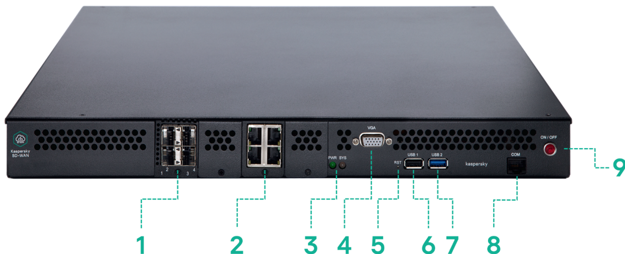
Рисунок 1.1. Передняя панель изделия
