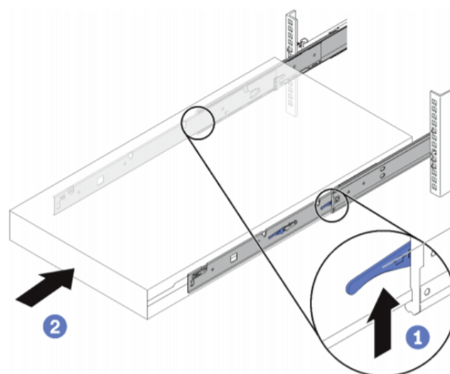
Рисунок 2.1. Установка изделия в стойку
