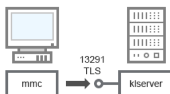
管理伺服器和主控台
