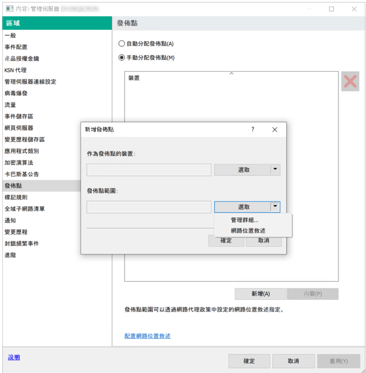
選取發佈點範圍
