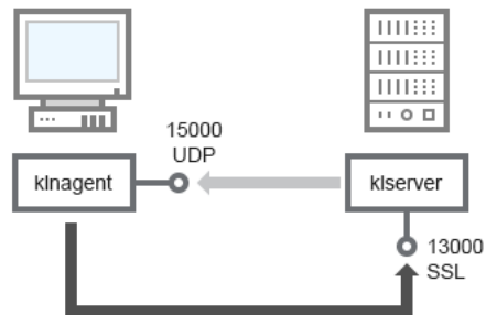
管理伺服器 and 用戶端裝置：管理安全應用程式、透過連接埠 13000 連線（建議）
