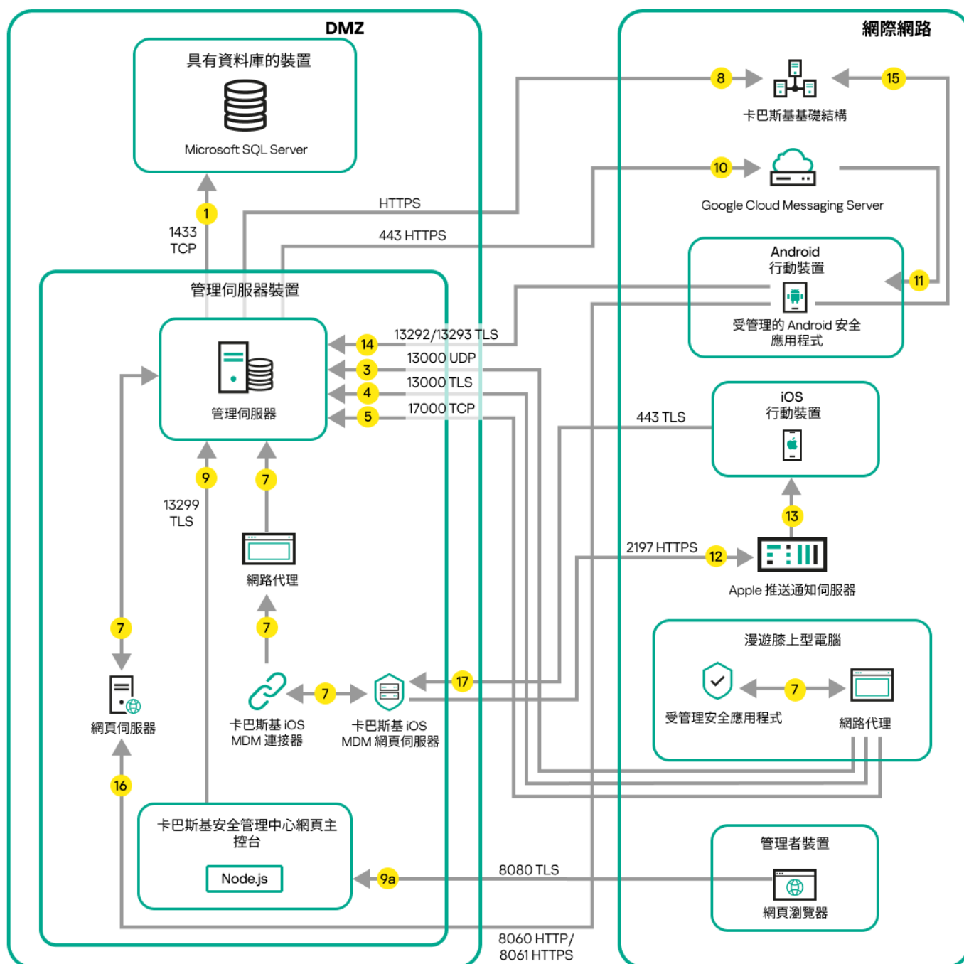
管理伺服器位於 DMZ、受管理行動裝置位於網際網路
