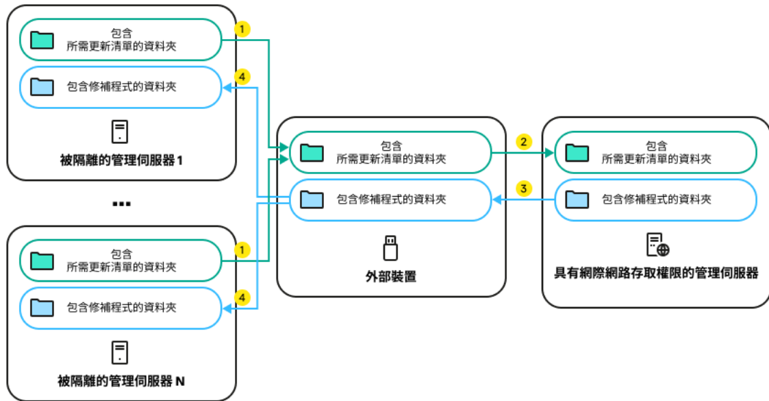
在具有網際網路存取權限的管理伺服器 and 隔離的管理伺服器之間傳輸修補程式和所需更新清單的過程
