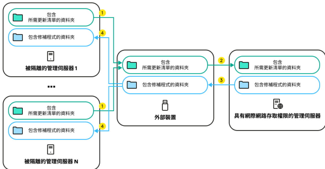
在具有網際網路存取權限的管理伺服器和隔離的管理伺服器之間傳輸修補程式和所需更新清單的過程
