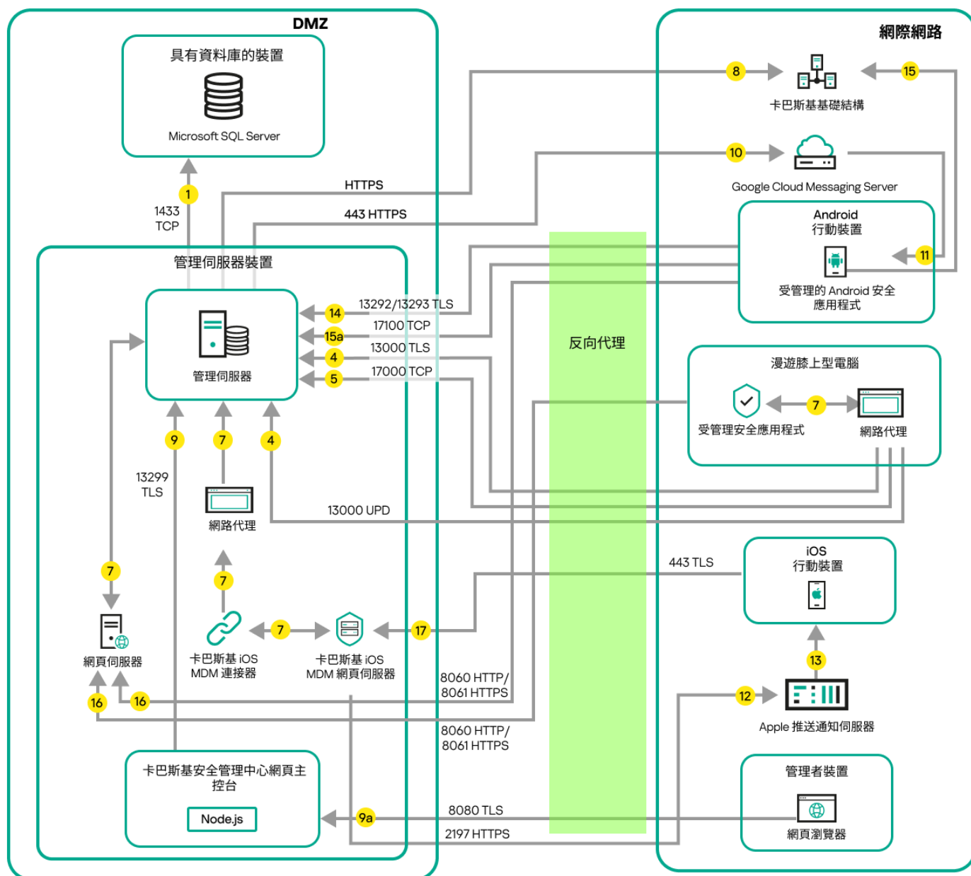
管理伺服器位於區域網路；受管理裝置透過反向代理連線到管理伺服器
