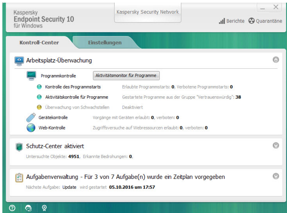
Programmhauptfenster
